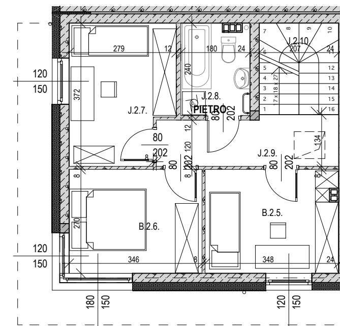
RZUT PIĘTRA
