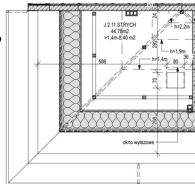
RZUT STRYCHU (strych do adaptacji po przeznaczeniu)
