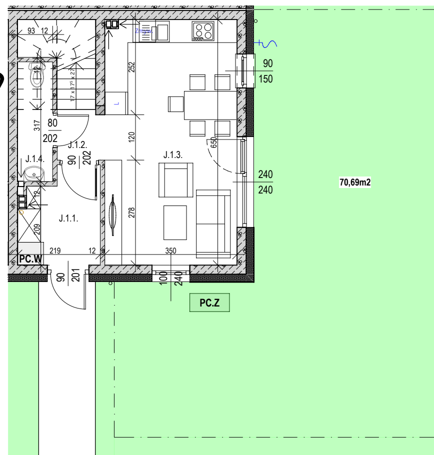
RZUT PARTERU
