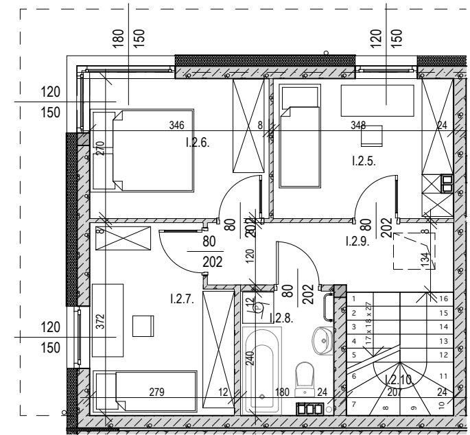
RZUT PIĘTRA
