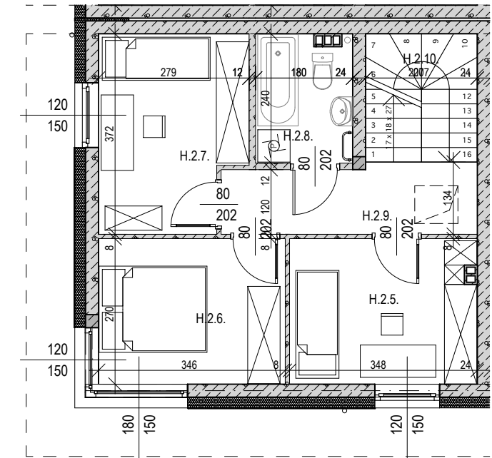
RZUT PIĘTRA
