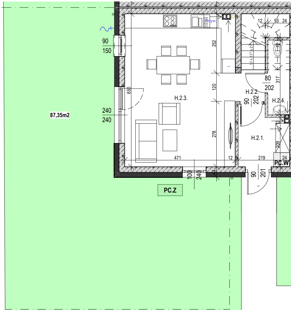
RZUT PARTERU
