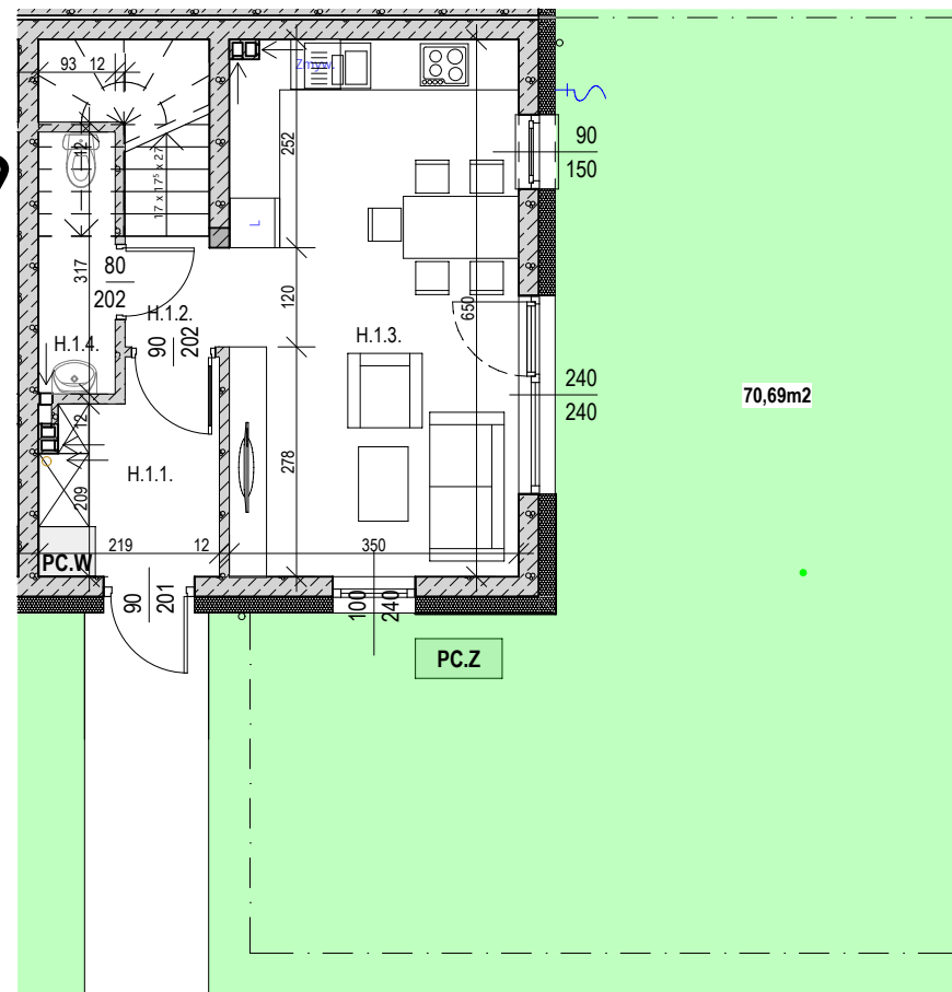
RZUT PARTERU
