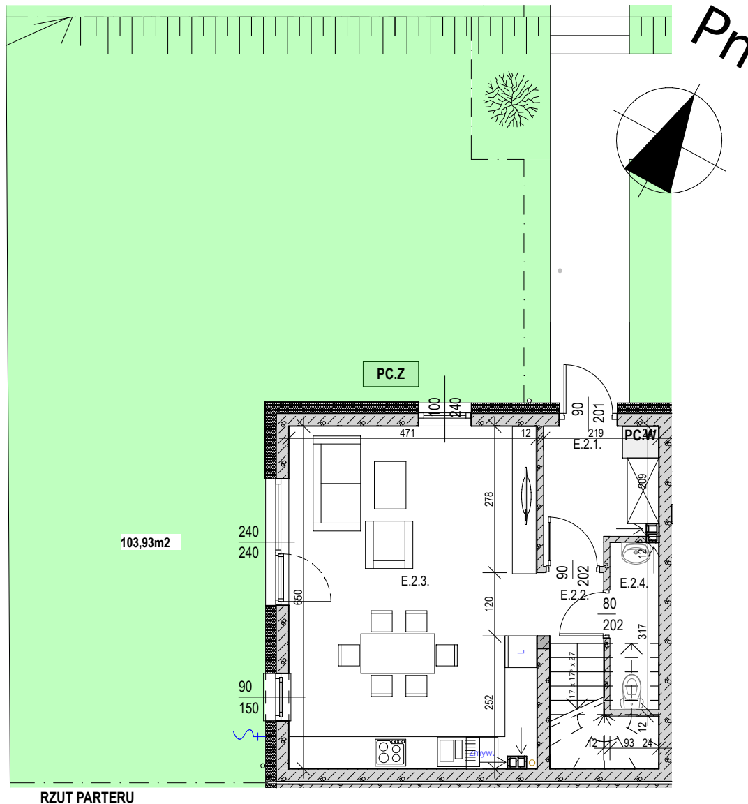
RZUT PARTERU
